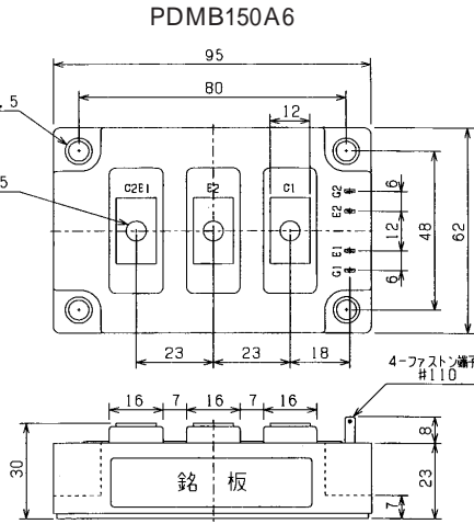
外形寸法図 OUTLINE DRAWING
