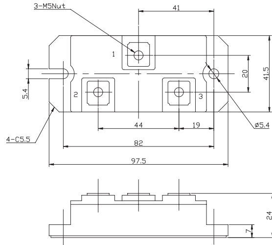
外形寸法図 OUTLINE DRAWING (単位 Dimension : mm)
