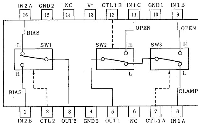
NJM2508D NJM2508M NJM2508V
