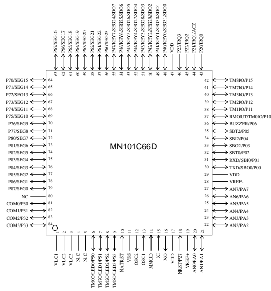
QFP084-P-1818E *Lead-free
