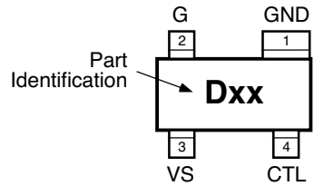
SOT-143 (M4)
