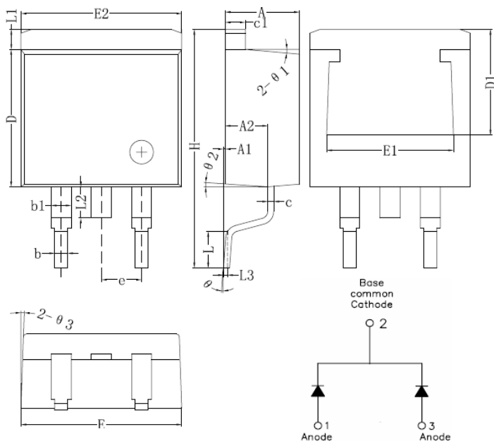
D 2 PAK
