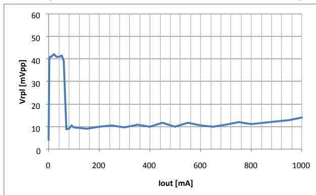
Vin=3.7V, Vout=1.5V
