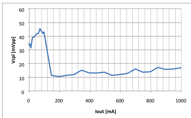
Vin=3.7V, Vout=2.5V
