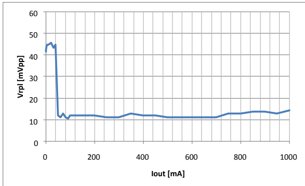
Vin=3.7V, Vout=1.5V
