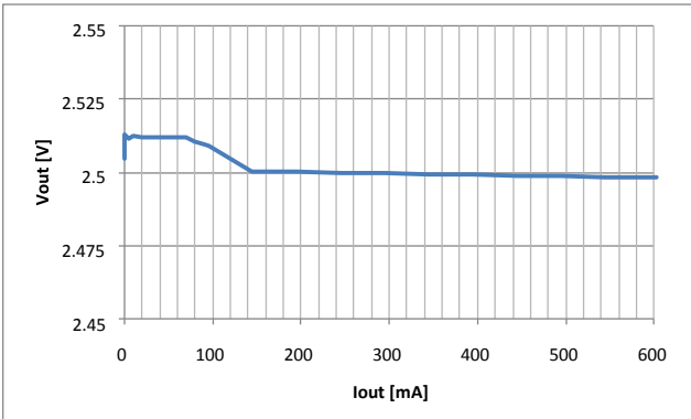
Vin=3.7V, Vout=2.5V
