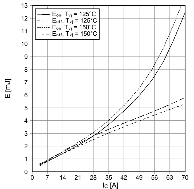
Schaltverluste IGBT-Wechselr. (typisch) switching losses IGBT-inverter (typical) E_{on} = f(I_c) , E_{off} = f(I_c) V_{GE} = \pm 15\text{ V} , R_{Gon} = 12\ \Omega , R_{Goff} = 12\ \Omega , V_{CE} = 600\text{ V}
