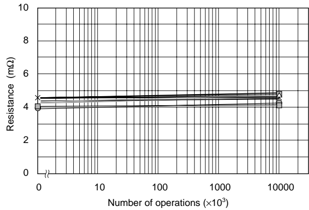
Contact Resistance (N.C contact)
