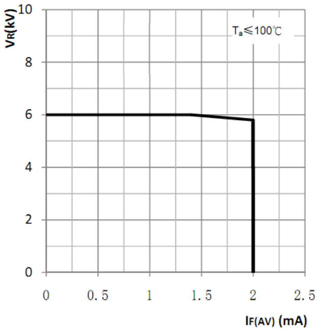
V_R - I_F (AV) Curve
