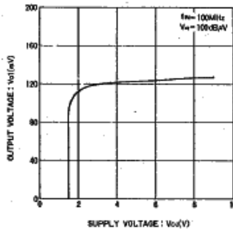
Fig.5 出力電圧1-電源電圧特性
