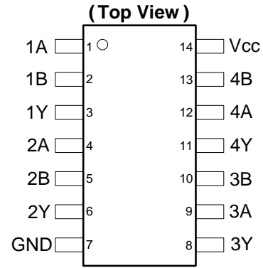
SO-14 / TSSOP-14
