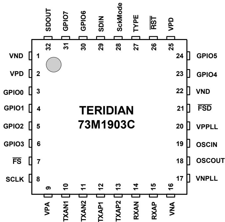
73M1903C QFN 32
