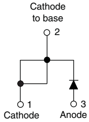
VS-60EPU06PbF
