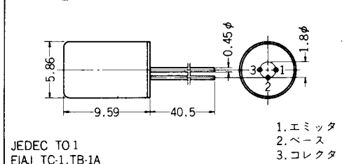
外形図-29
